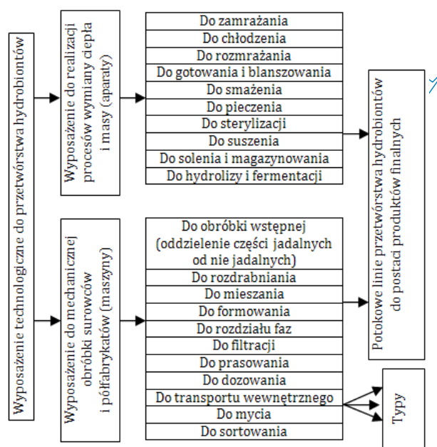
Rys. 4. Ogólna klasyfikacja wyposażenia stosowanego w przetwórstwie ryb i innych hydrobiontów według jednostkowych procesów
